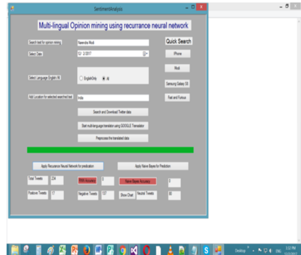
Fig. 10. Apply RNN
